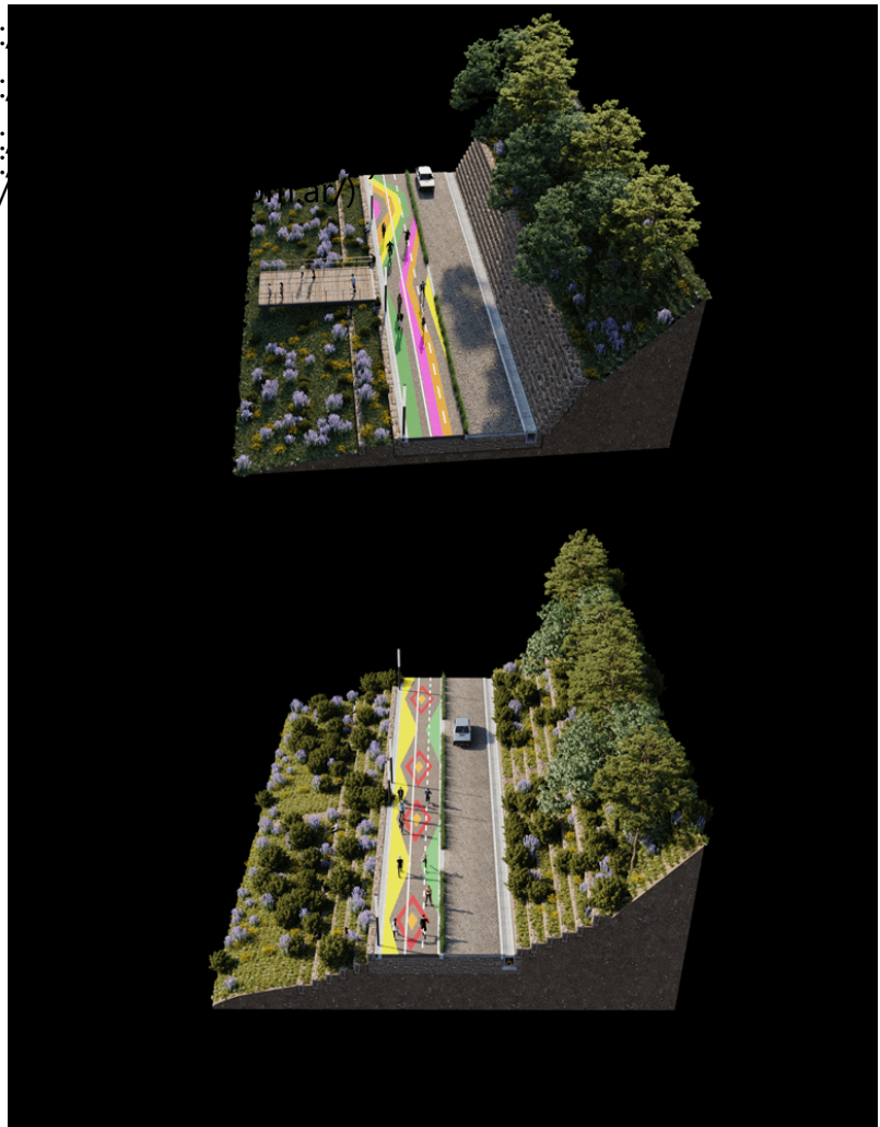
(https://oficinaurbana.com.ar/project/parque-lineal-metropolitano-la-paz-el-alto-bolivia/70_22_la-paz_axonometrica-corte-tipo-k/)
